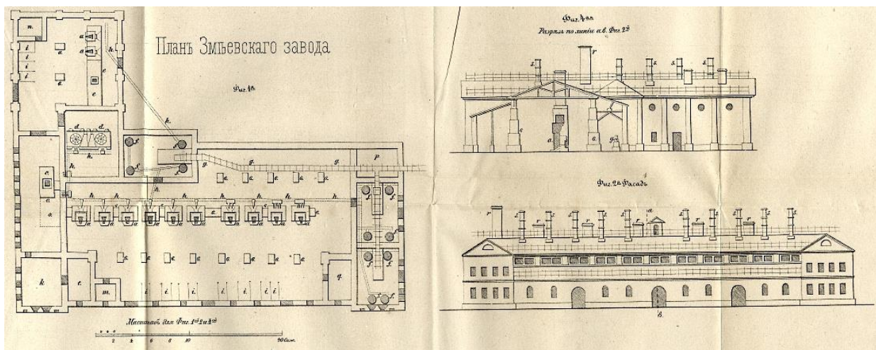
Ранний план Змеиногорского сереброплавильного завода. Горный журнал за 1884 год.
