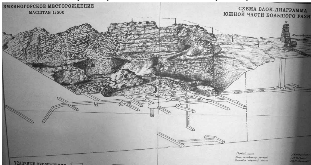
Схема южной части большого разноса, составленная в начале XX века М.Ф. Розеном.
