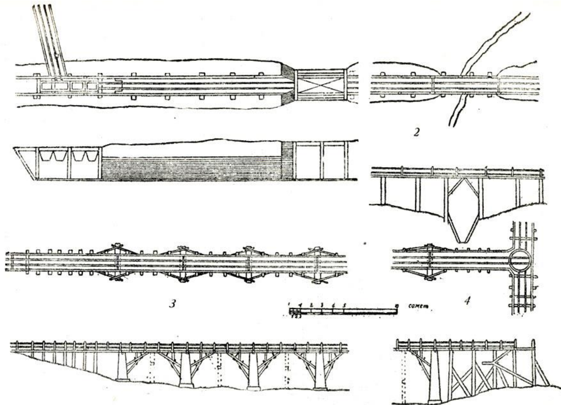
Рис. 73. Первая рельсовая дорога в России, сооруженная П. К. Фроловым в 1806—1809 годах.—Новосибирский областной государственный архив. 1 — начальная часть дороги с бункерами и концом переносной дороги (А); 2 — малый мост; 3 — начало виадука; 4 — конец виадука, поворотный круг и начало „флагелей“ (ответвлений).
