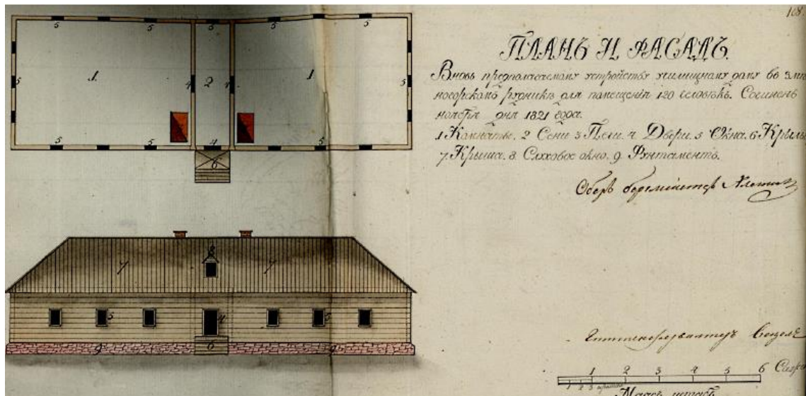
План и фасад Змеиногорской горнозаводской школы 1821 год. (ГААК. Ф.2. Оп.1. Д.2056. Л.1051)
